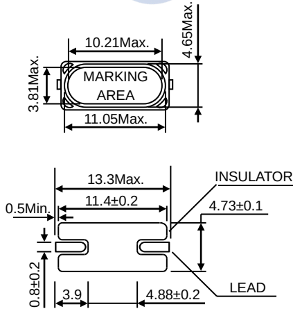
HC-49X 系列
